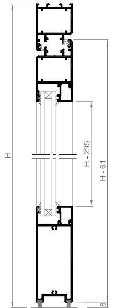
SECCIÓN B-B'
