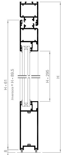
SECCIÓN B-B'
