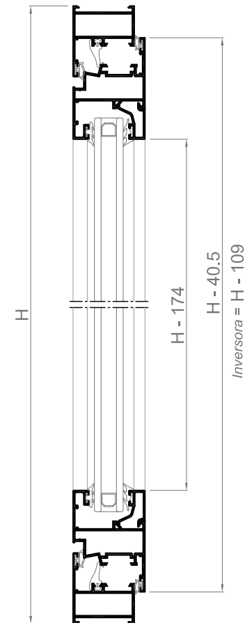
Sección B-B'
