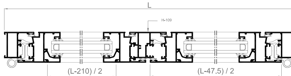
Sección A-A'
