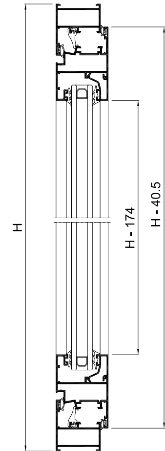
Sección B-B'
